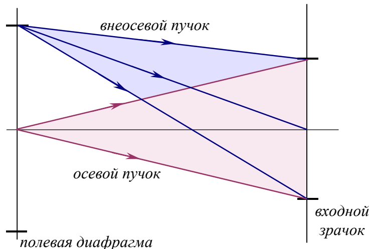
Рис.7.2.3. Полевая диафрагма.
