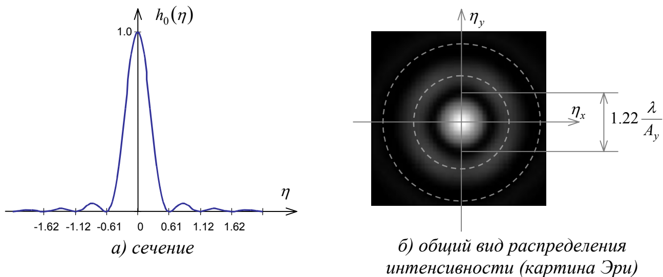
Рис.9.3.1. Функция рассеяния точки в отсутствие aberrаций.
