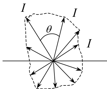
Рис.2.3.1. Диаграмма силы света.
