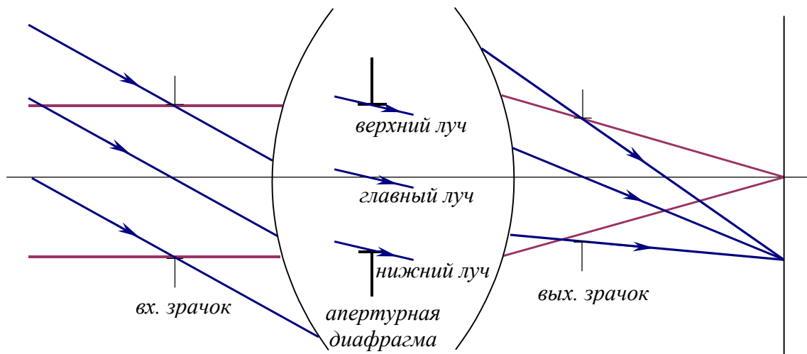
Рис.7.2.2. Внеосевой пучок.
