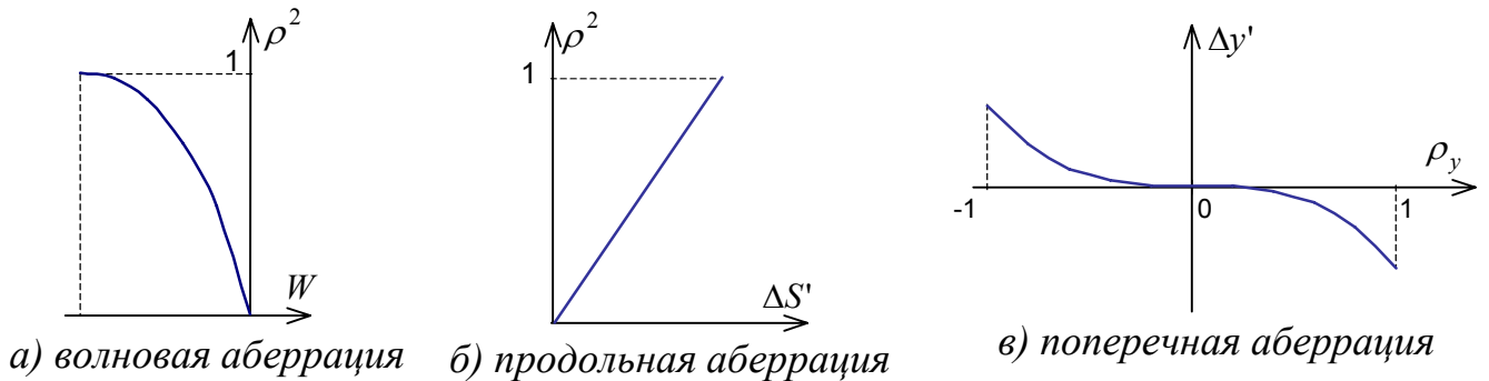
Рис.8.2.4. Графики aberrаций для сферической aberrации 3 порядка.
