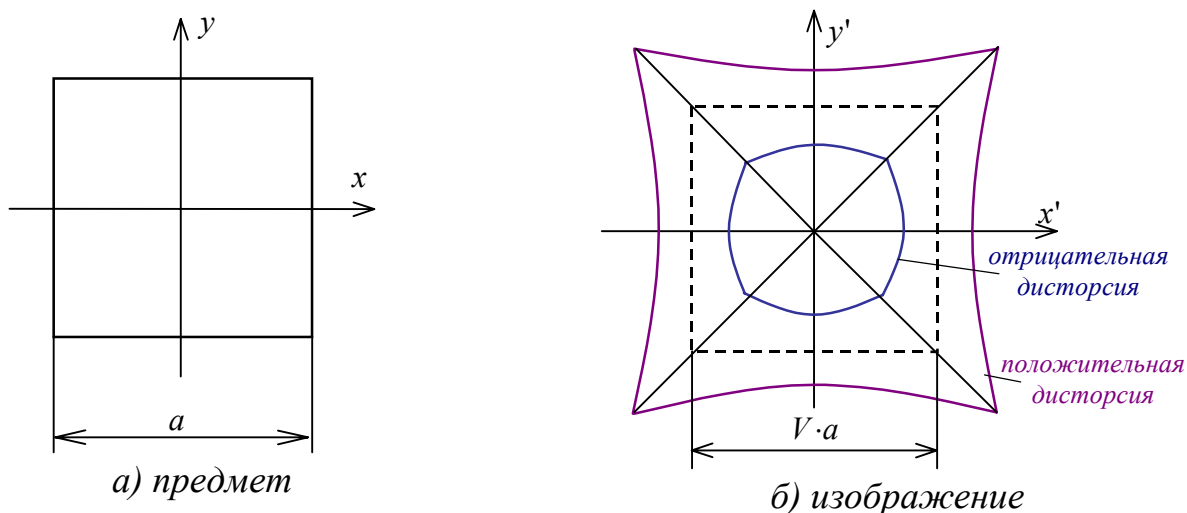
Рис.8.2.18. Дисторсия.
