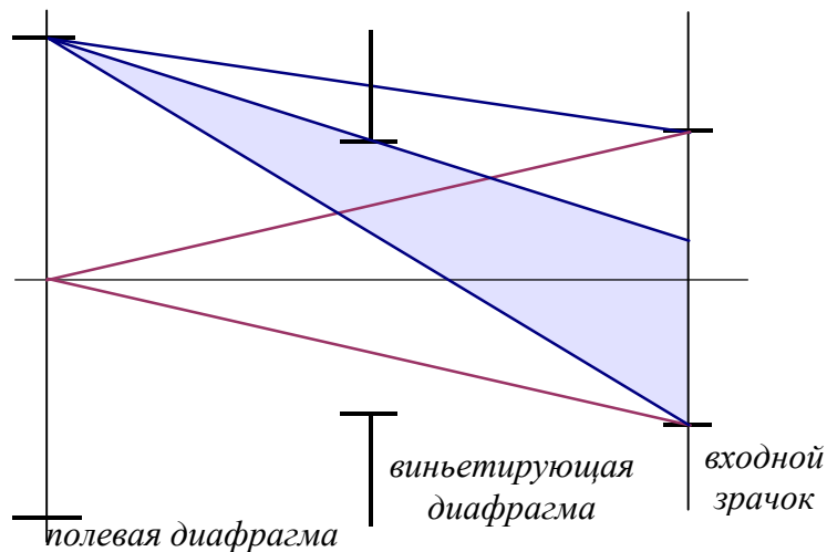
Рис.7.2.4. Виньетирование.
