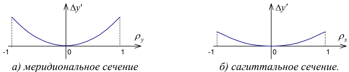
Рис.8.2.9. Поперечные абберации при коме 3 порядка.
