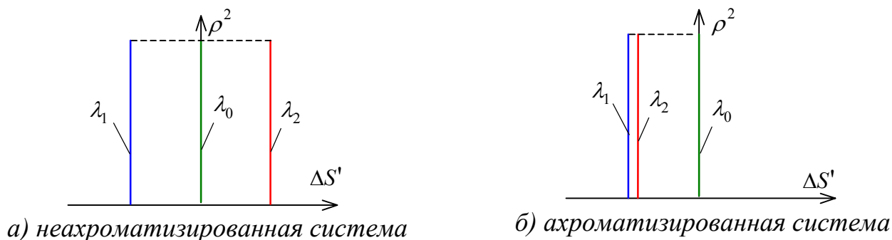
Рис.8.3.5. Продольный хроматизм первого порядка.
