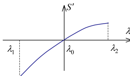
Рис.8.3.2. График зависимости положения изображения от длины волны.
