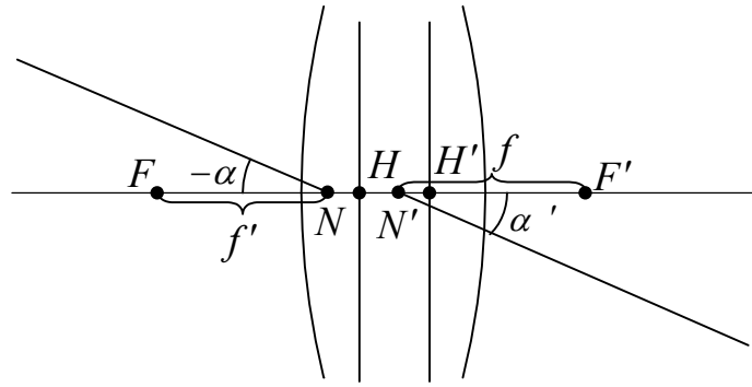
Рис.5.3.2. Узловые точки.
