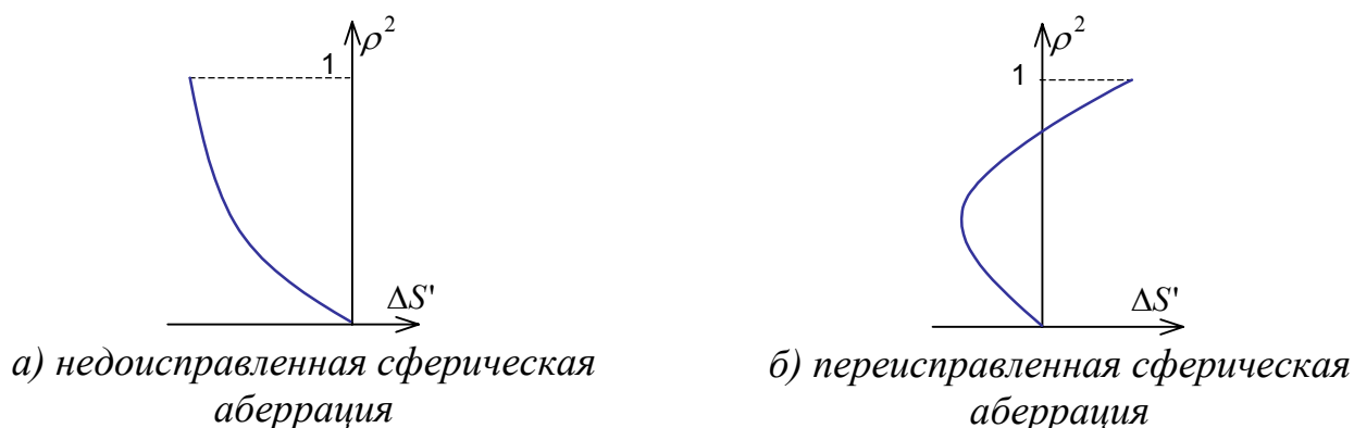
Рис.8.2.6. Графики коррекции сферической aberrации.
