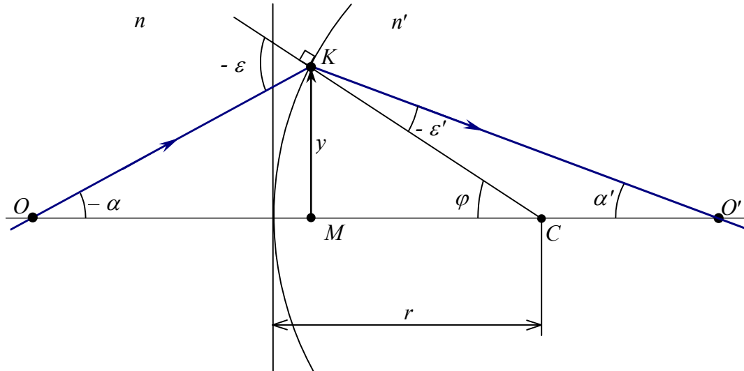
Рис.6.2.5. Преломляющая поверхность.
