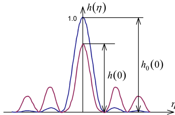
Рис.9.5.3. Число Штреля.
