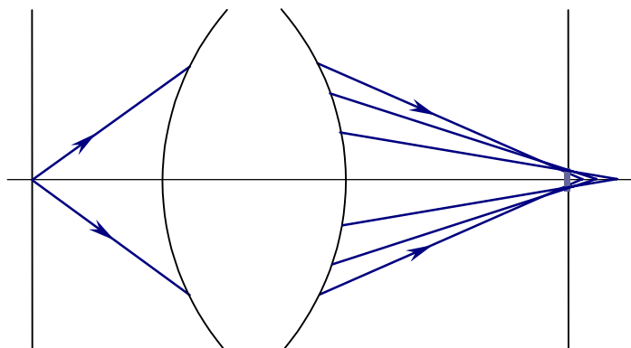
Рис.8.2.3. Сферическая aberrация.
