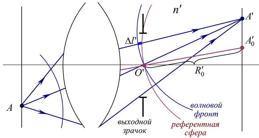
Рис.8.1.5. Волновая aberrация.
