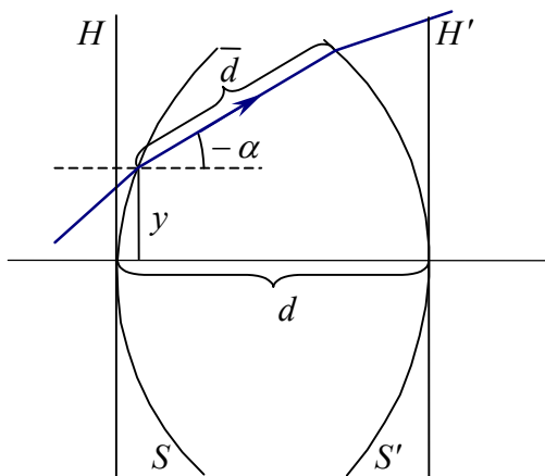
Рис.7.1.1. Ход реального луча.
