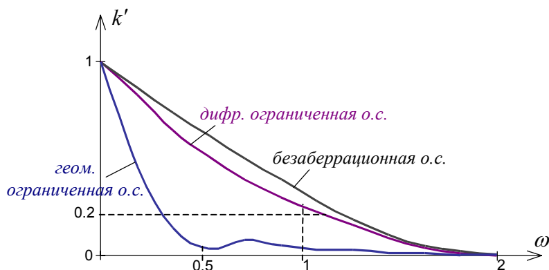
Рис.9.5.4. Влияние aberrаций на ЧКХ.
