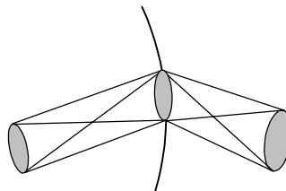
Рис.4.3.5. Инвариант Штраубеля.
