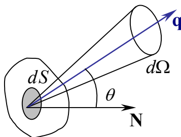
Рис.2.1.4. Энергетическая яркость.
