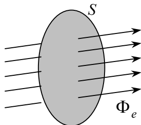
Рис. 2.1.1. Поток излучения.
