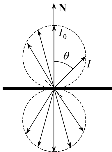
Рис. 2.3.3. Плоский ламбертовский излучатель.
