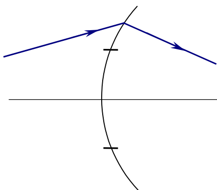
Рис.7.1.5. Реальный луч проходит за краем диафрагмы.
