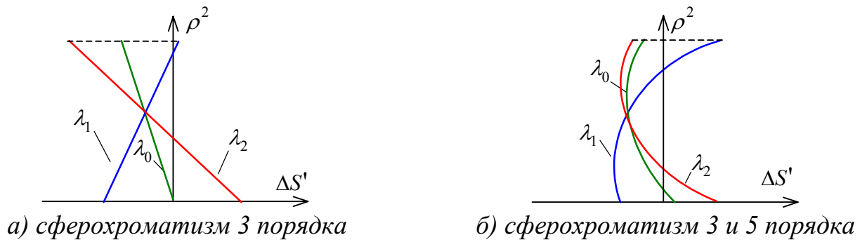
Рис.8.3.8. Сферохроматизм в присутствии aberrаций 3 и 5 порядков.
