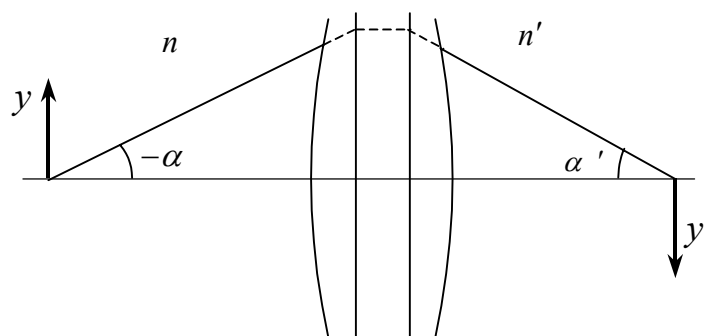
Рис.5.3.4. Величины, которые связывает инвариант Лагранжа-Гельмгольца.
