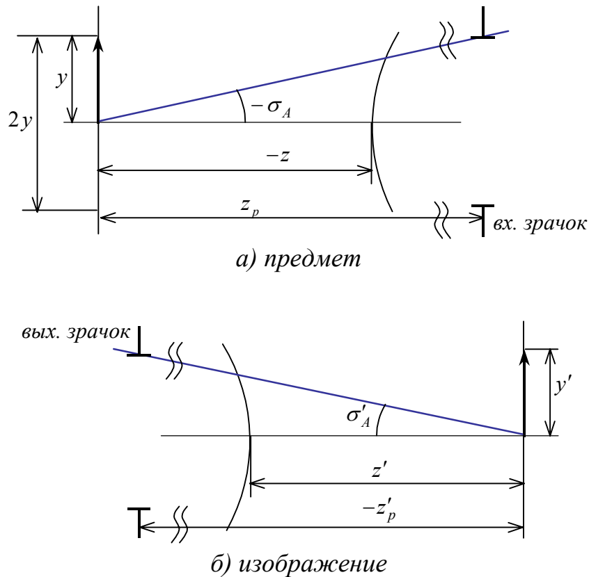
Рис.7.3.1. Предмет и изображение ближнего типа.
