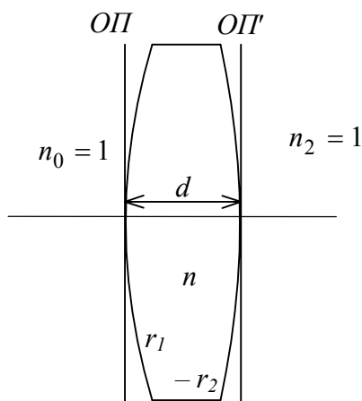
Рис.6.3.4. Линза в воздухе.
