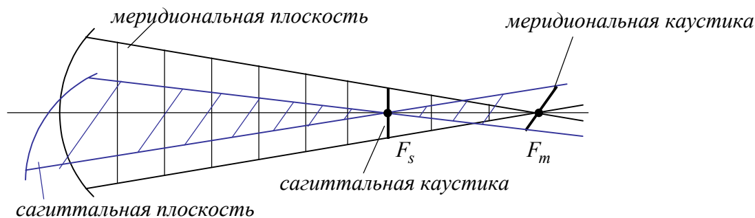
Рис.4.4.4. Астигматический пучок.
