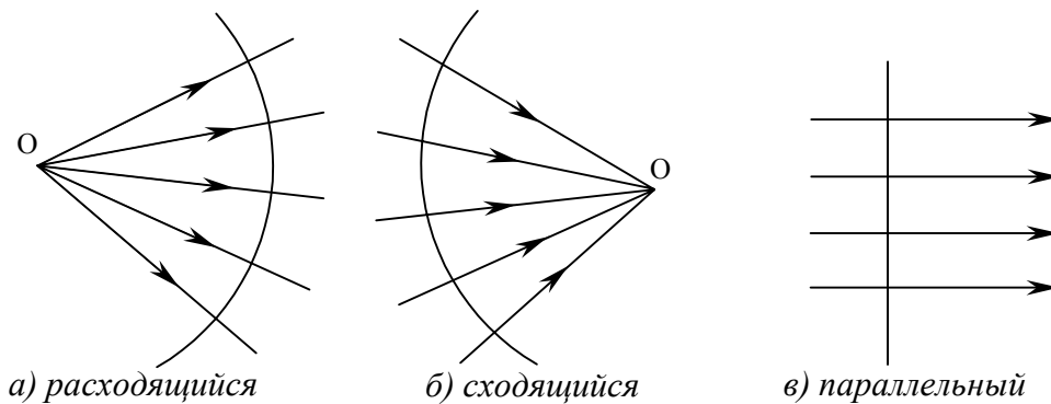
Рис.4.4.1. Пучки лучей.
