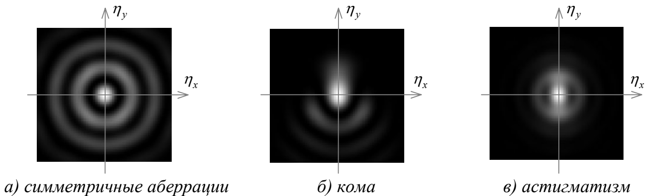
Рис.9.5.2. Картины Эри для aberrаций различных типов.
