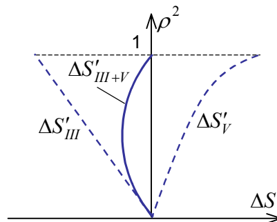
Рис.8.2.5. Взаимокомпенсация сферической aberrации 3 и 5 порядков.
