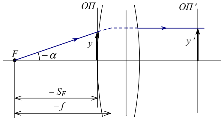
Рис.6.2.2. Схема для нахождения элементов B и D матрицы преобразования.
