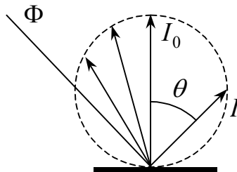
Рис.2.5.1. Ламбертовское рассеяние.
