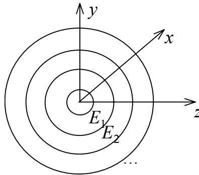
Рис.1.4.3. Сферические волны.
