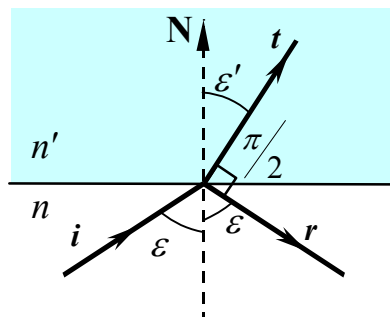
Рис.3.3.1. Угол Брюстера.
