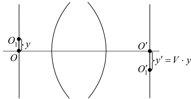
Рис.9.1.1. Условие изопланатизма.
