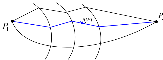
Рис.4.3.2. Принцип Ферма.
