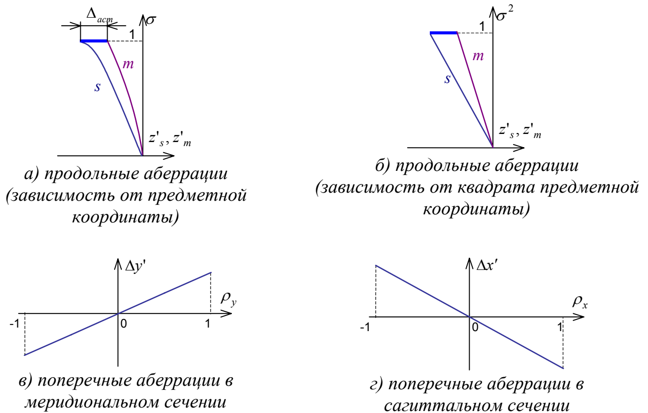
Рис.8.2.13. Астигматизм 3 порядка (продольные и поперечные aberrации).
