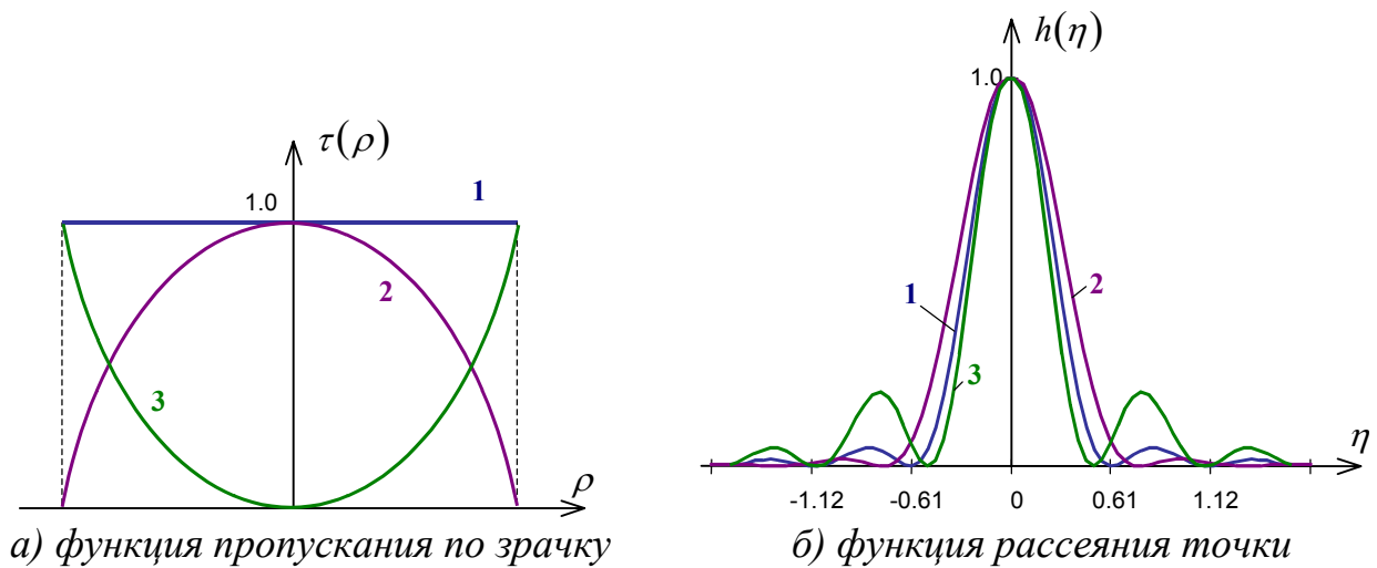
Рис.9.3.2. Влияние неравномерности пропускания по зрачку на ФРТ.
