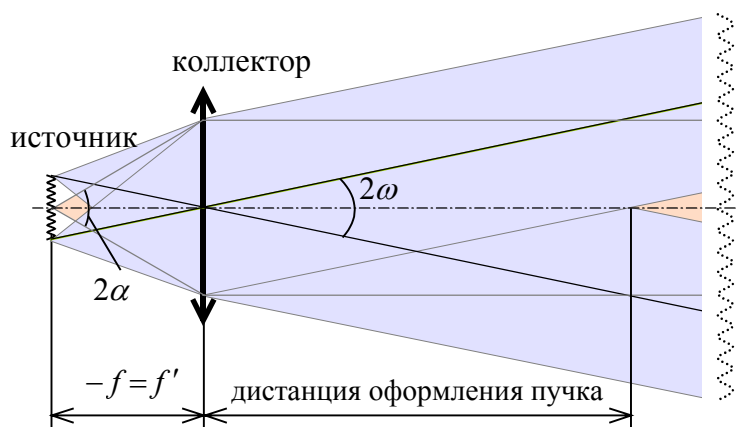
Рис. 7.7. Схема прожектора.
