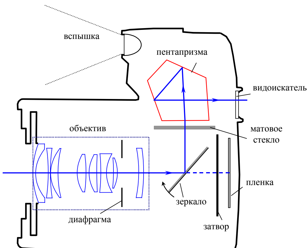
Рис. 4.4. Зеркальный фотоаппарат.
