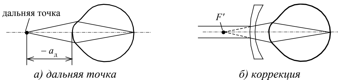
Рис. 2.7. Коррекция близорукости.
