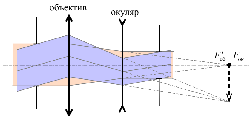
Рис. 5.5. Схема Галилея.
